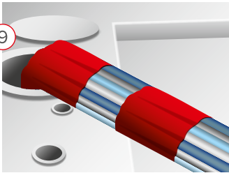
Marcado de cables, encintado y protección
